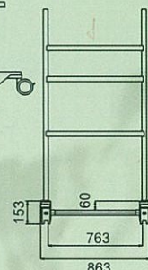
TYPE3 MW151 863mm(w)x1515mm(H)700MM(D) 1.基本框架 2.把手固定平盤X1 3.固定平盤X2 4.鍵盤台X1(擴充) 5.電源組X1(擴充)
