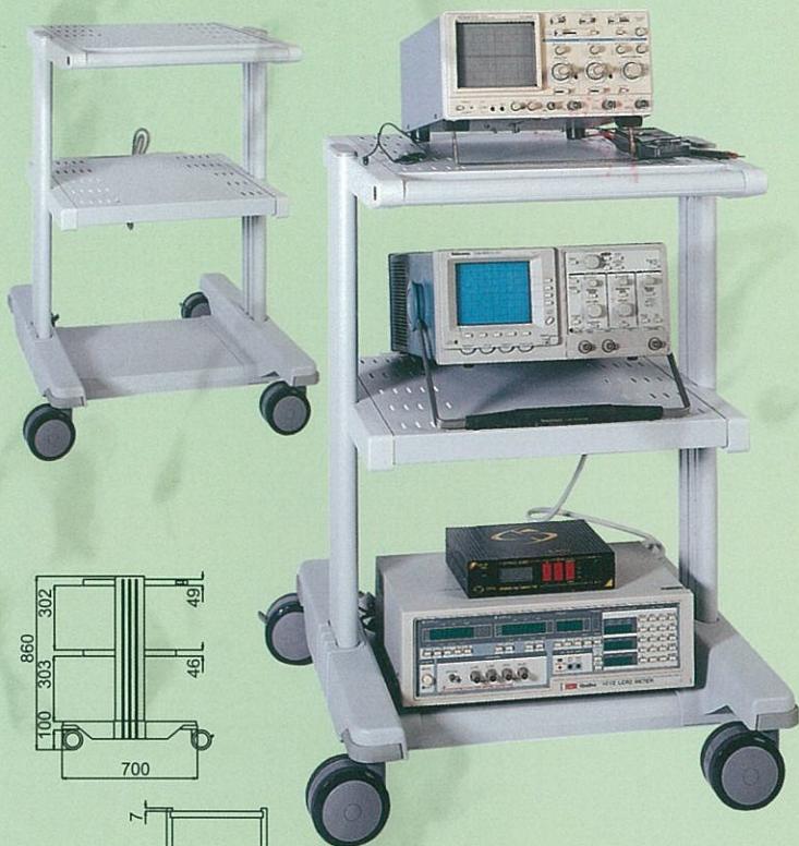
TYPE1 MW86 696mm(w)x860mm(H)700MM(D) 1.基本框架 2.固定平盤X1 3.把手固定平盤X1 4.電源組X1(擴充)
