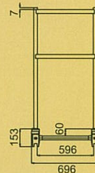
TYPE2 MW112 696mm(w)x1120mm(H)700MM(D) 1.基本框架 2.固定平盤X1 3.鍵盤台X1(擴充) 4.抽屜X1(擴充) 5.把手固定平盤X1 6.電源組X1(擴充)
