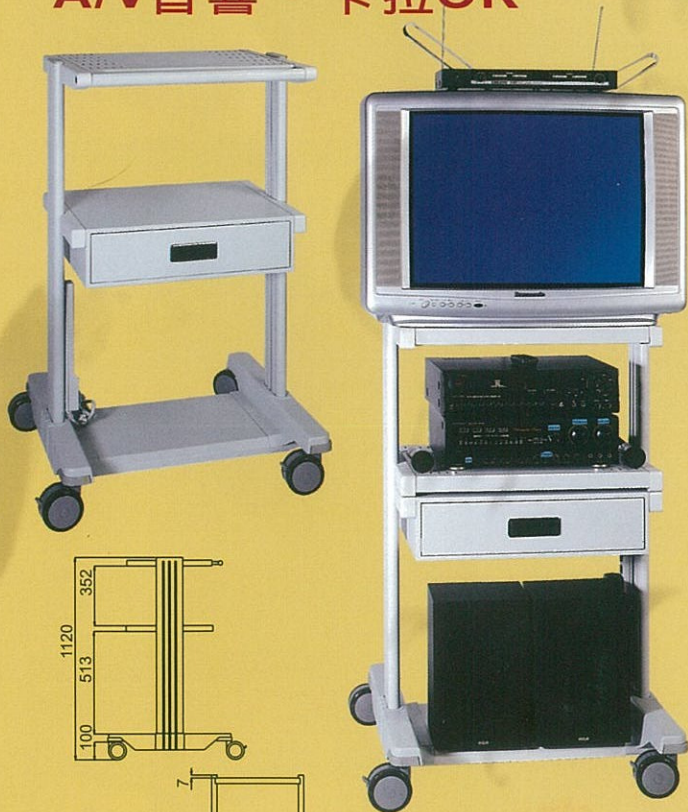
TYPE2 MW112 696mm(w)x1120mm(H)700MM(D) 1.基本框架 2.固定平盤X1 3.抽屜X1(擴充) 4.電源組X1(擴充) 5.把手固定平盤X1 6.電源組(擴充)
